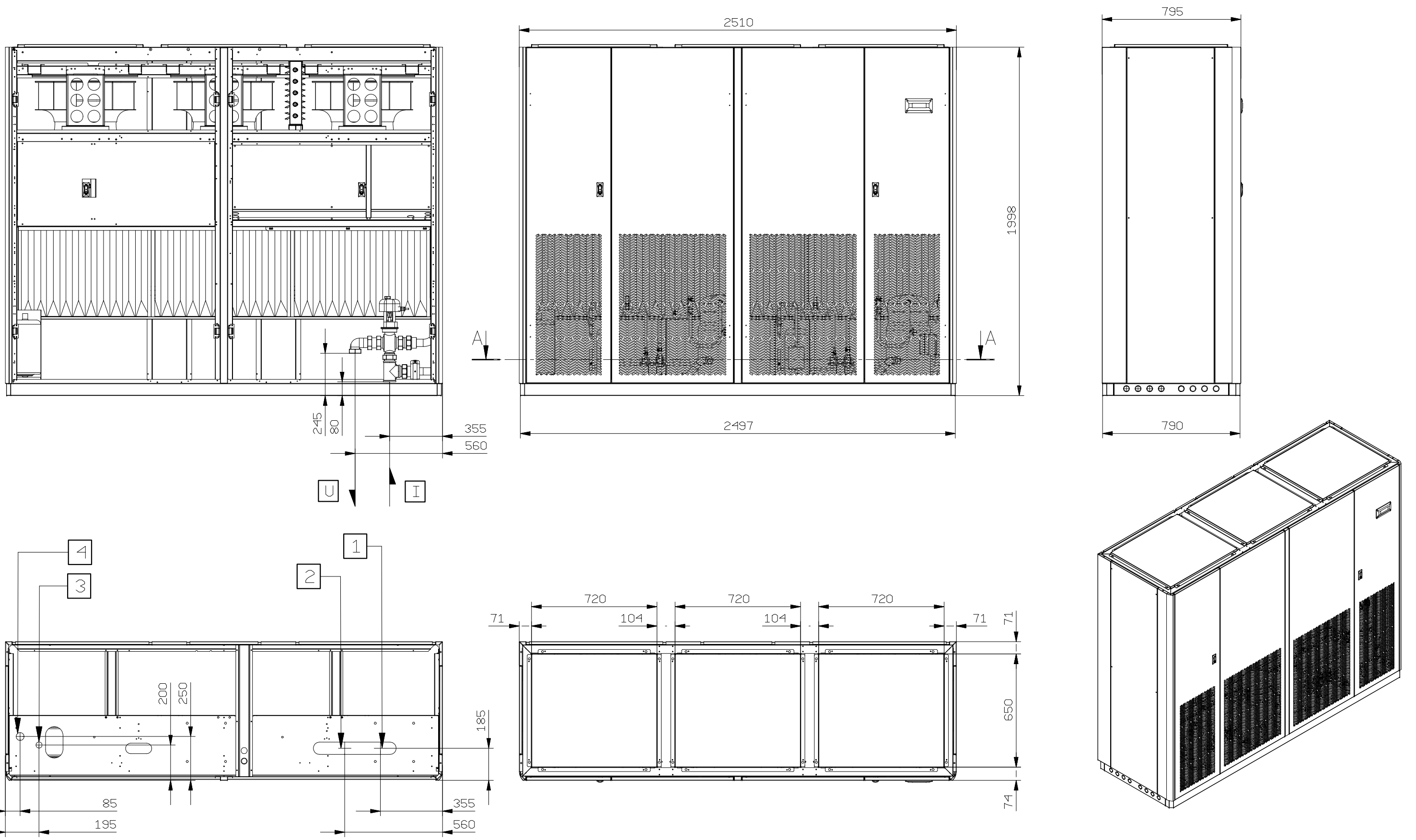
section A-A
