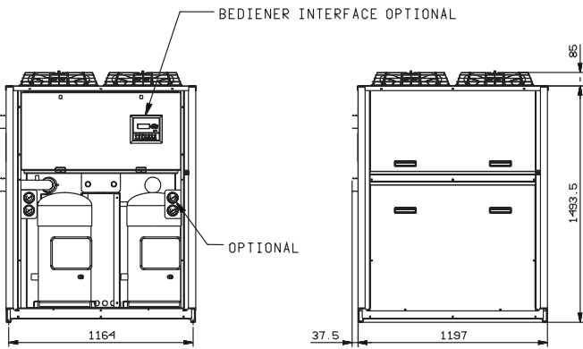
VORDERANSICHT
