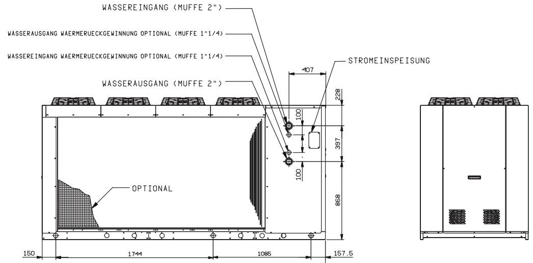
SEITENANSICHT
